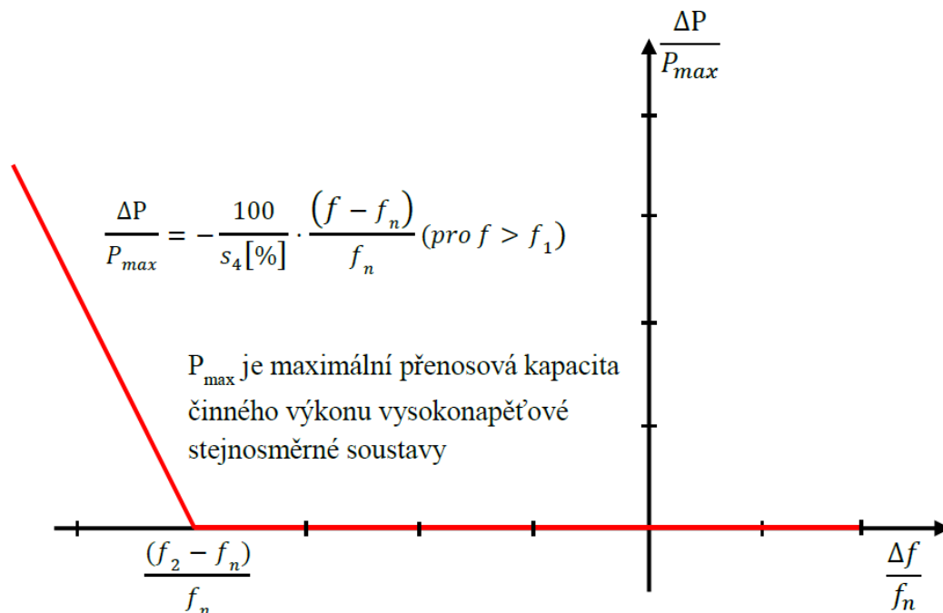
Obr. 5: Schopnost frekvenční odezvy činného výkonu u vysokonapěťových stejnosměrných soustav v omezeném frekvenčně závislém režimu při podfrekvenci. \Delta P je změna činného výkonu na výstupu z vysokonapěťové stejnosměrné soustavy, v závislosti na provozních podmínkách snížení importovaného výkonu nebo zvýšení exportovaného výkonu. f_n je jmenovitá frekvence střídavé soustavy nebo soustav, ke které (kterým) je vysokonapěťová stejnosměrná soustava připojena, a \Delta f je změna frekvence střídavé soustavy nebo soustav, ke které (kterým) je vysokonapěťová stejnosměrná soustava připojena. Při podfrekvencích, kdy f je nižší než f_2 , musí vysokonapěťová stejnosměrná soustava zvýšit činný výkon na výstupu podle statiky s_4 .
