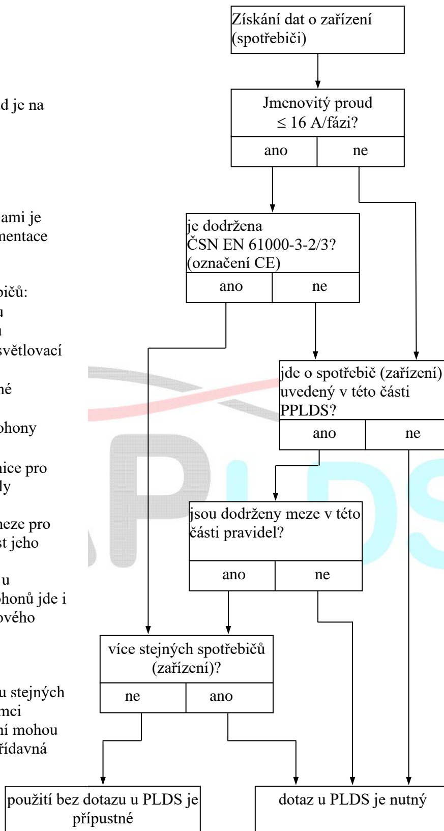
Obr. 1 Schéma po posuzování přístrojů/zařízení se zřetelem na elektromagnetickou kompatibilitu EMC)
