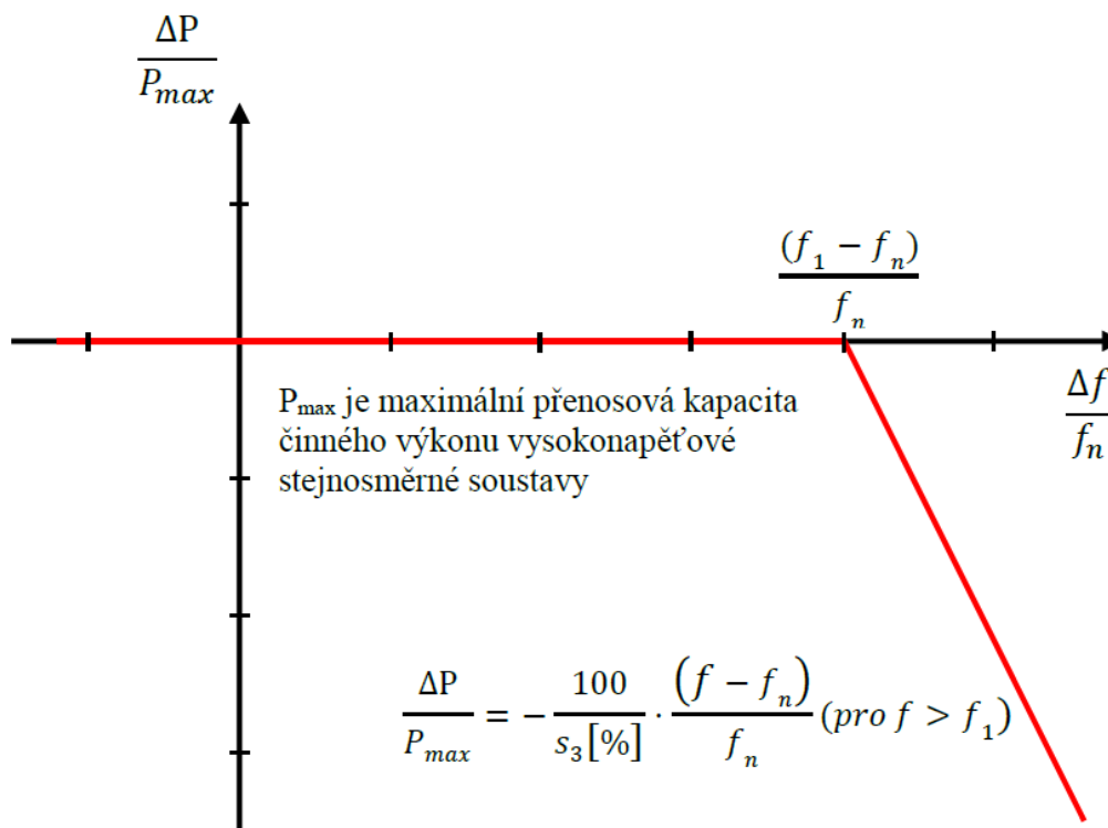
Obr. 4: Schopnost frekvenční odezvy činného výkonu u vysokonapěťových stejnosměrných soustav v omezeném frekvenčně závislém režimu při nadfrekvenci. \Delta P je změna činného výkonu na výstupu z vysokonapěťové stejnosměrné soustavy a v závislosti na provozních podmínkách buď snížení importovaného výkonu, nebo zvýšení exportovaného výkonu. f_n je jmenovitá frekvence střídavé soustavy nebo soustav, ke které (kterým) je vysokonapěťová stejnosměrná soustava připojena, a \Delta f je změna frekvence střídavé soustavy nebo soustav, ke které (kterým) je vysokonapěťová stejnosměrná soustava připojena. Při nadfrekvencích, kdy f je vyšší než f_1 , musí vysokonapěťová stejnosměrná soustava snížit činný výkon podle nastavení statiky s_3 .
